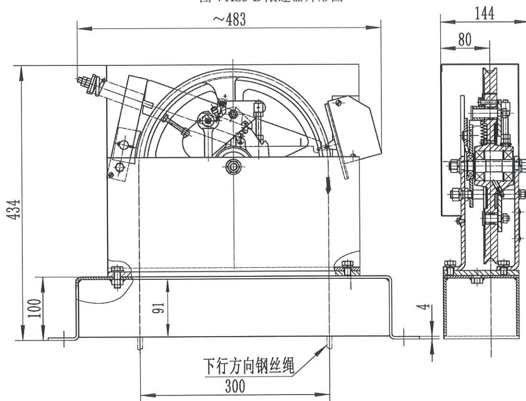
图 5 XS18B 限速器外形图
