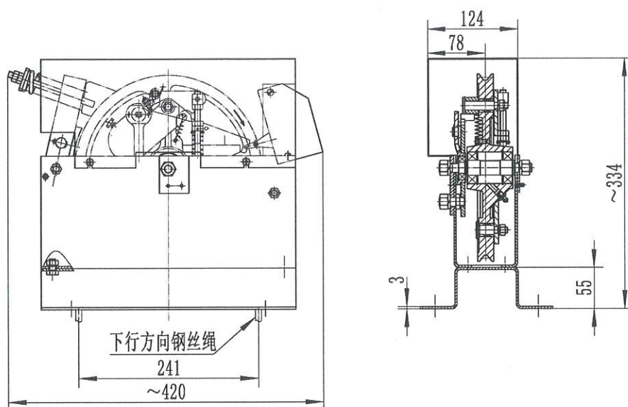
图 2 XS3 限速器外形图
