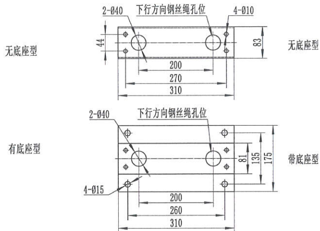
图 7 XS3C 型限速器底座安装参数
