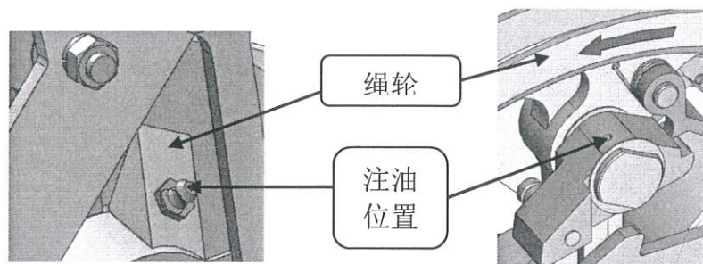
图 12 注油示意图
