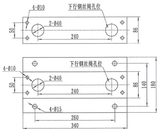
图 6 XS3 型限速器底座安装参数
