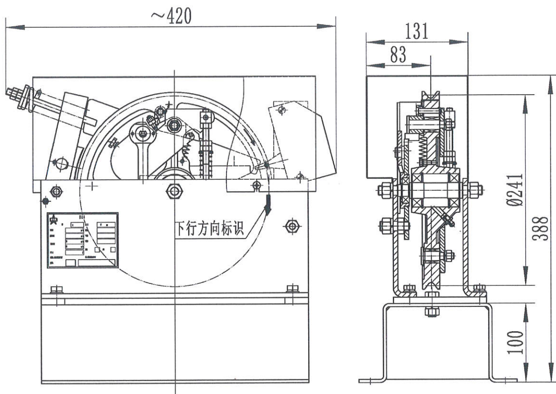
图 4 XS3-B 限速器外形图
