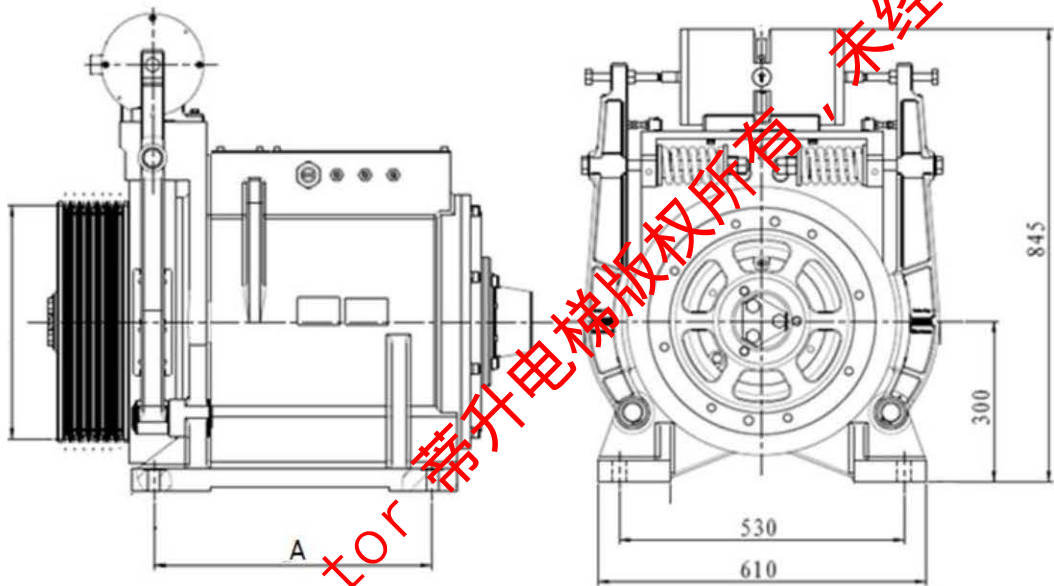
图 3-1 PMS300 曳引机（不含附件）的外形尺寸图
