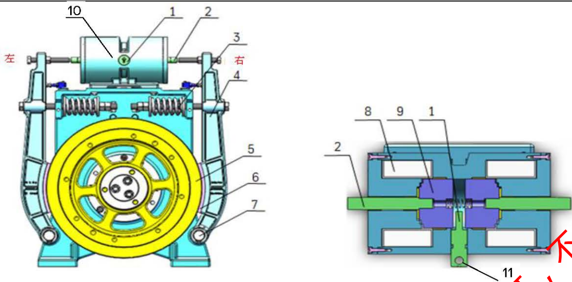
1) 释放轴 2) 推杆 3) 制动弹簧 4) 制动臂组件 5) 制动轮 6) 制动片 7) 制动臂销轴 8) 线圈 9) 衔铁 10) 电磁铁 11) 释放轴孔 注：推杆 2 和衔铁 9 组成衔铁组件。
